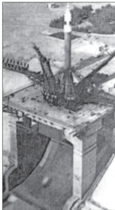
• Первая ракета Р-7 на старте.
